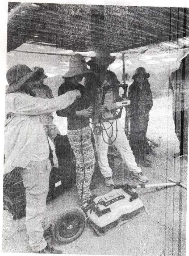
Foto 4. GPR
